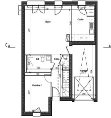
Rez-de-chaussée
